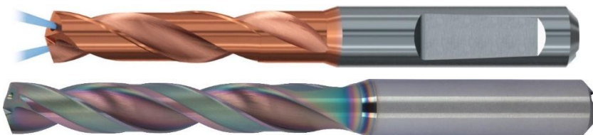
Bild 3 + Bild 4: Die EMUGE InoxDrill und SteelDrill Spiralbohrer sind in den Längen 3 x D und 5 x D in den Durchmessern von 3 bis 20 mm erhältlich.
